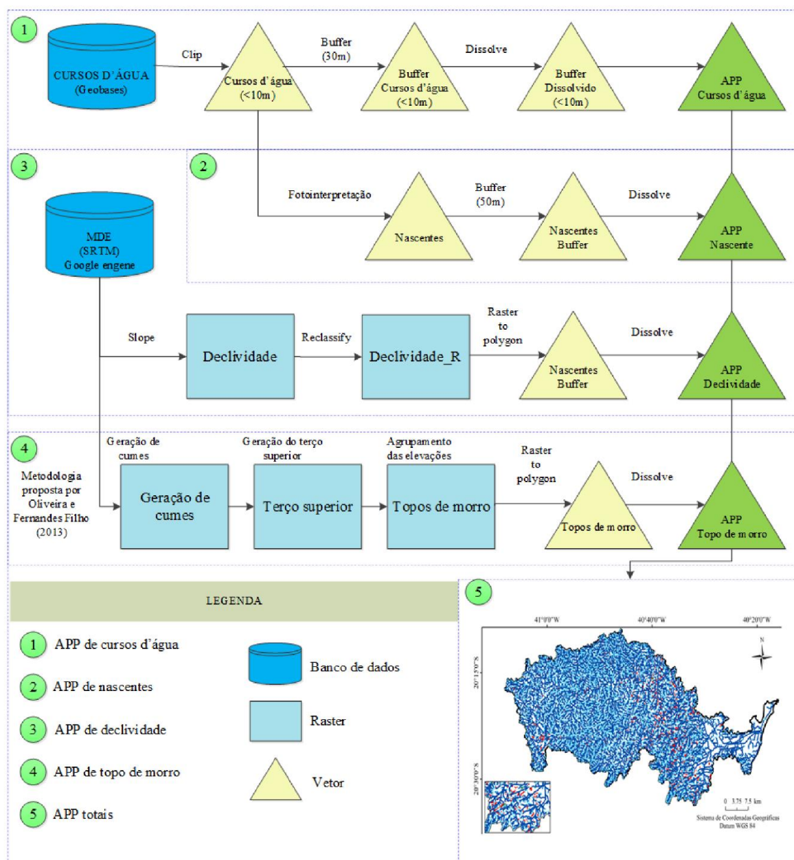
Figura 4 - Fluxograma contendo a metodologia utilizada para delimitação da APP na bacia hidrográfica do rio Jucu, de acordo com a legislação
